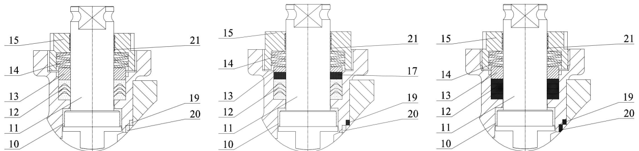
NP(Nut, PTFE)
